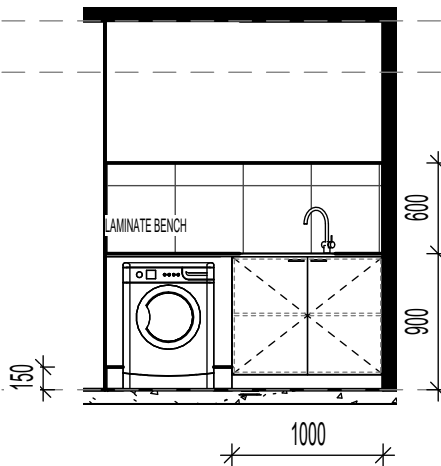
LAUNDRY 1 : 50
