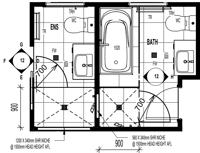
ENSUITE & BATHROOM FLOOR PLAN 1 : 50
