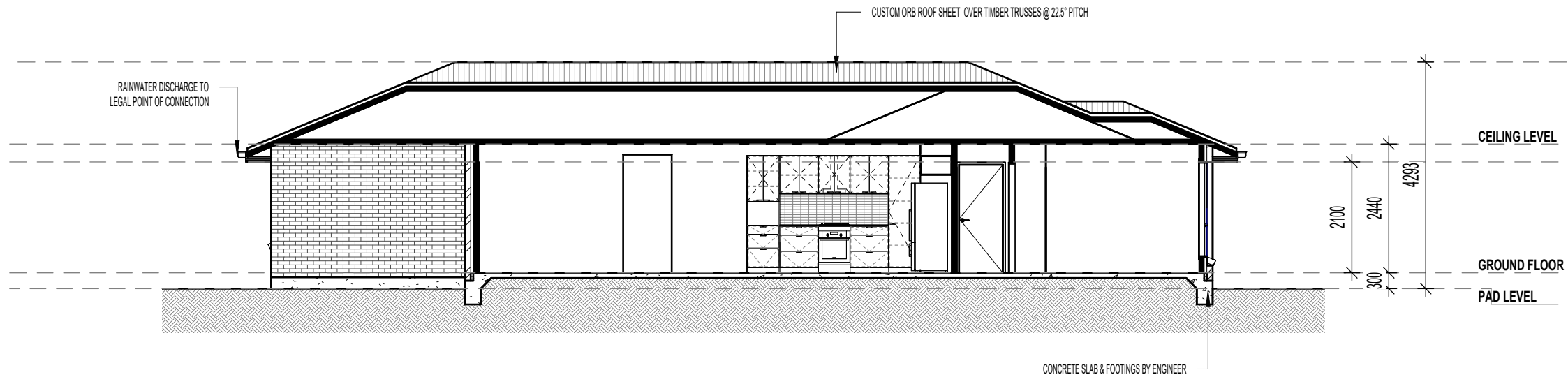
SECTION S1 1 : 100
