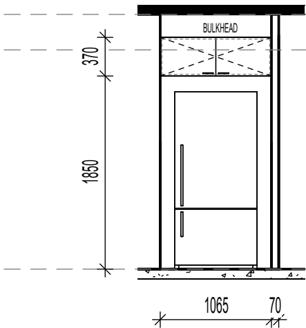
C 1 : 50
