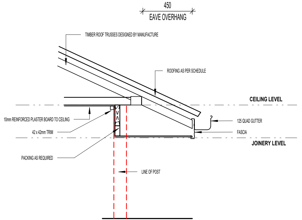
TYP. ALFRESCO EAVE DETAIL 1 : 20
