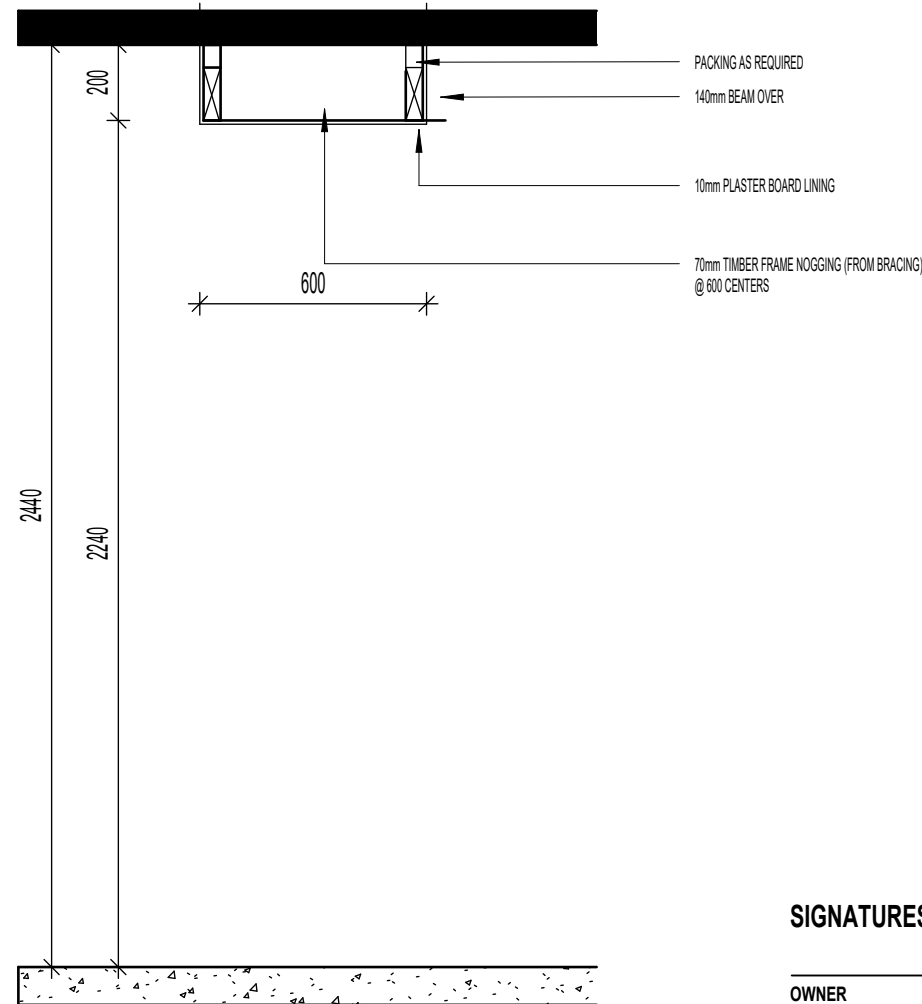
TYP. HALLWAY DETAIL 1 : 20
